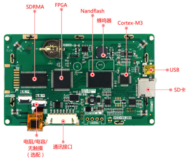
图 1-4 硬件配置图
