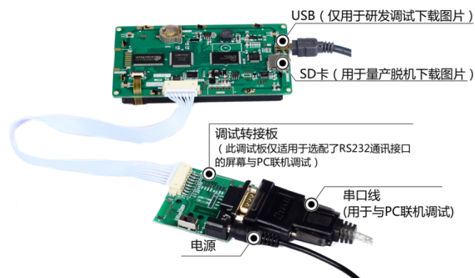
图 1-5 调试工具图
